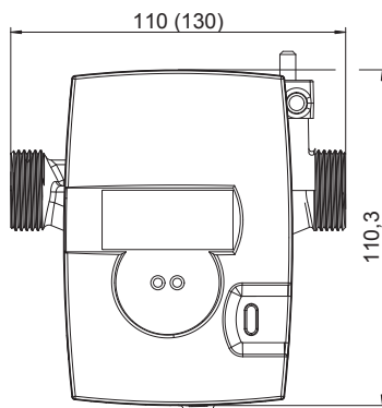
Draufsicht
